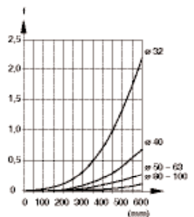
Отклонение (мм)
