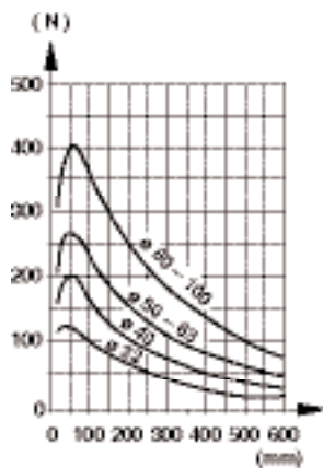
Нагрузочная способность
