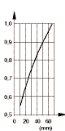
Корректирующий фактор
